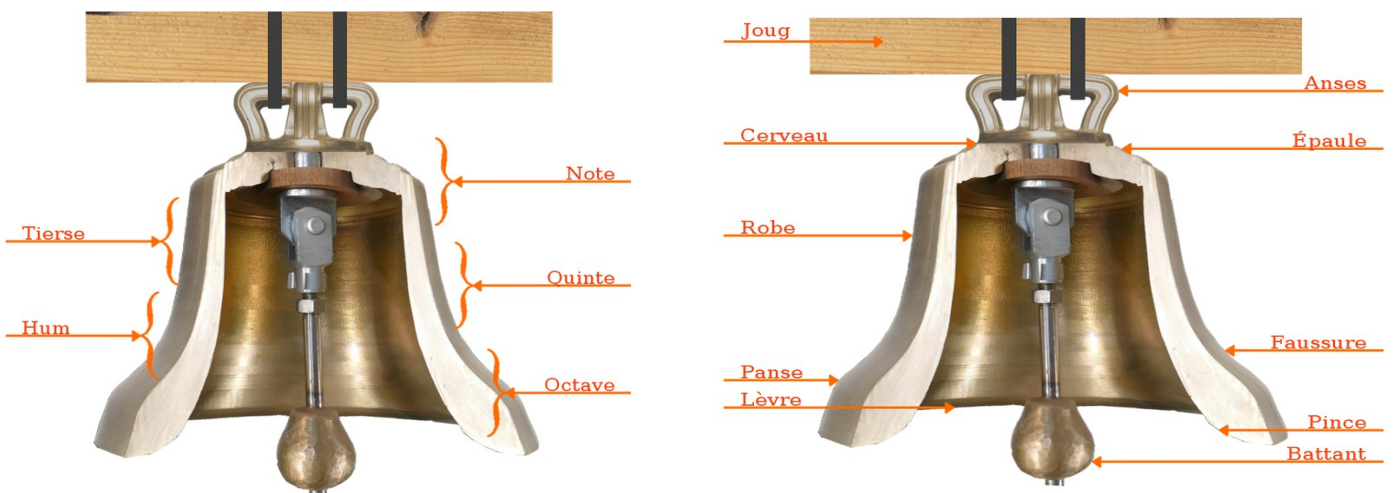
▲ Les différentes parties d'une cloche photo 1 ▲
